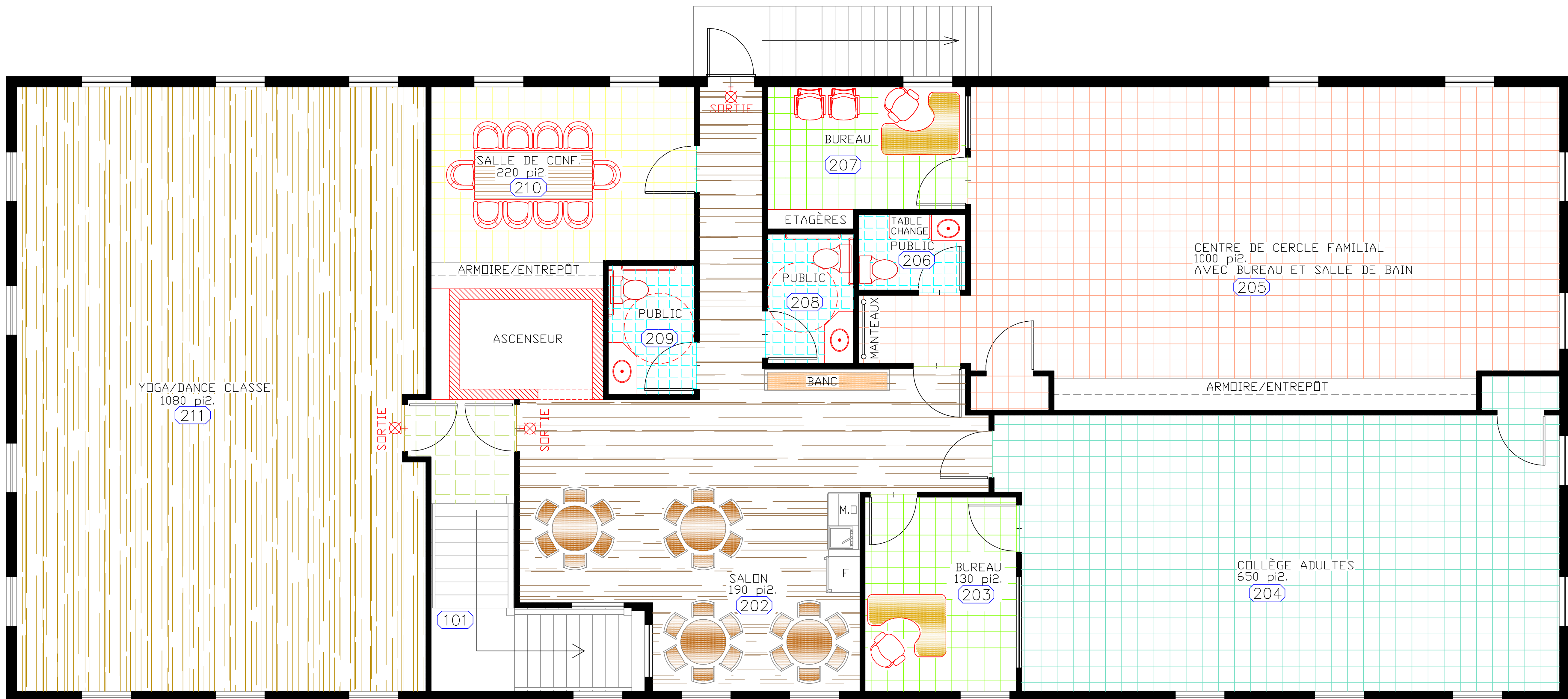
PLAN DU DEUXIEME PLANCHER
