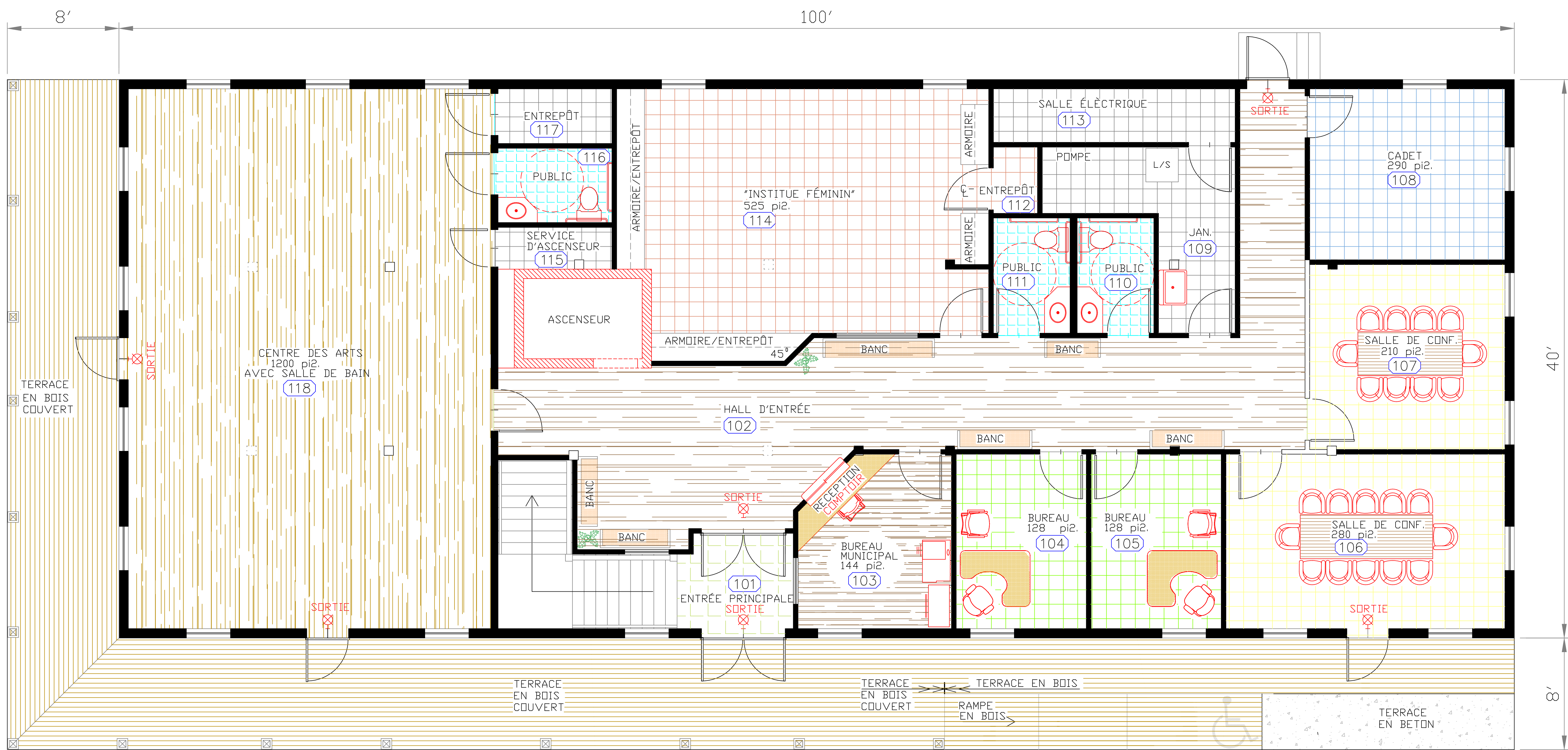
PLAN DU PREMIER PLANCHER
